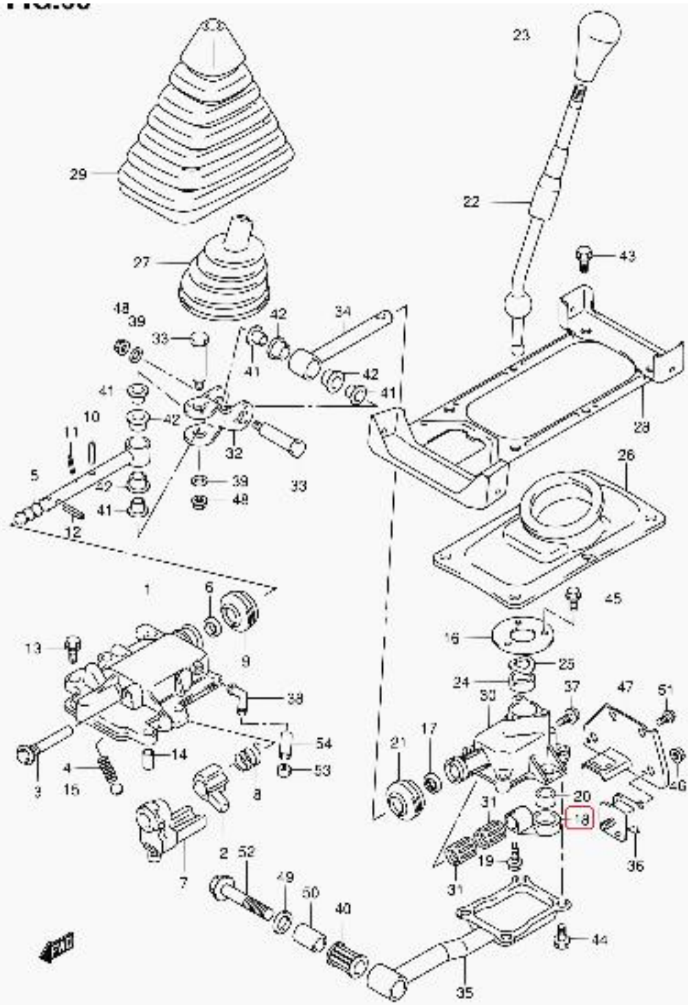
SN413V-2 E22 066 GEAR SHIFT CONTROL (VT SN413V)
