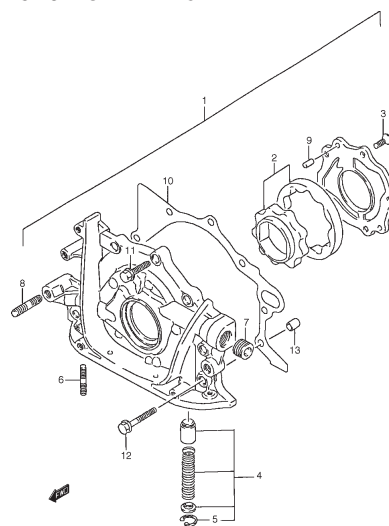
FIG. 6 BOMBA DE ACEITE
