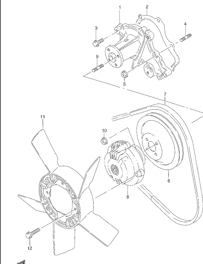
FIG. 18 BOMBA DE AGUA
