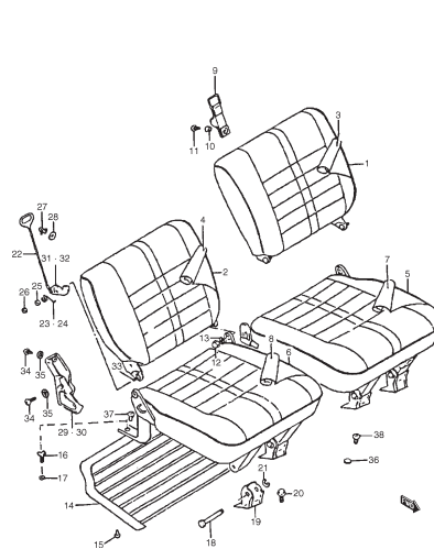
FIG. 95 ASIENTO TRASERO
