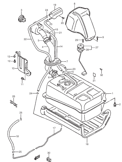
FIG. 93 DEPOSITO COMBUSTIBLE
