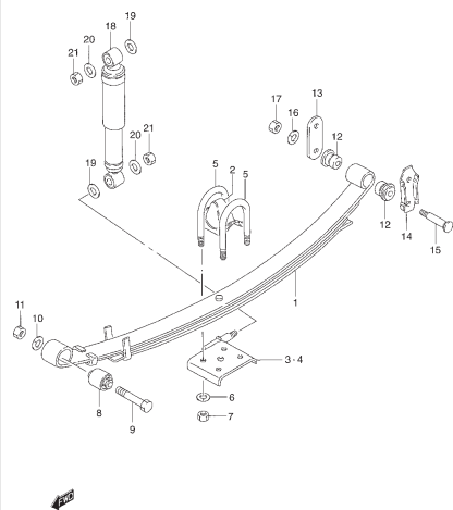
FIG. 49 SUSPENSION TRASERA
