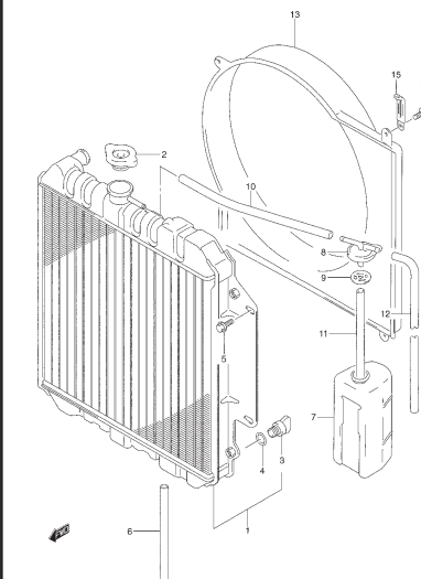
FIG. 19 RADIADOR
