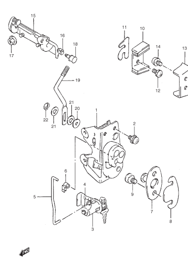
FIG. 91 CERRADURA PUERTA TRASERA (V)
