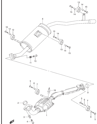
FIG. 16 SISTEMA DE ESCAPE
