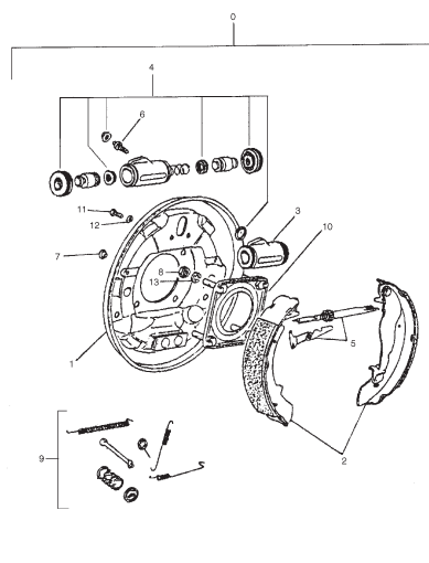
FIG. 62 FRENO TRASERO
