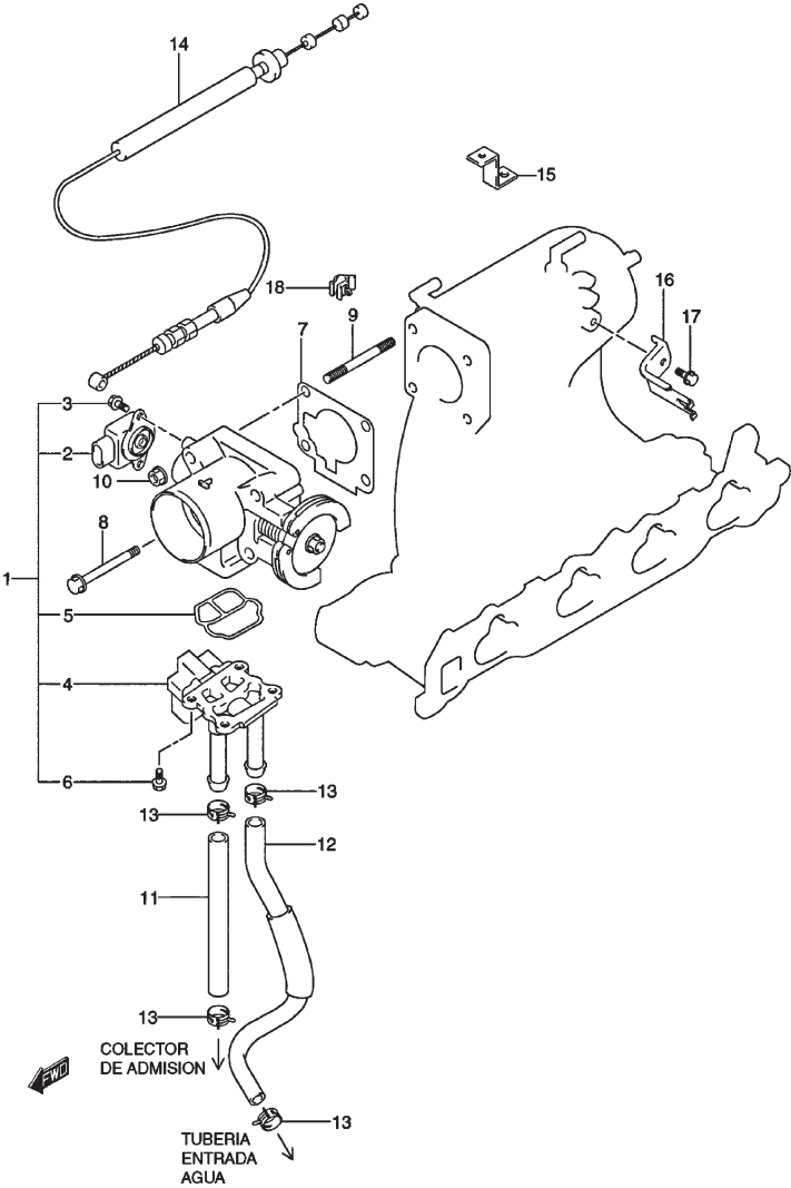
FIG.12
