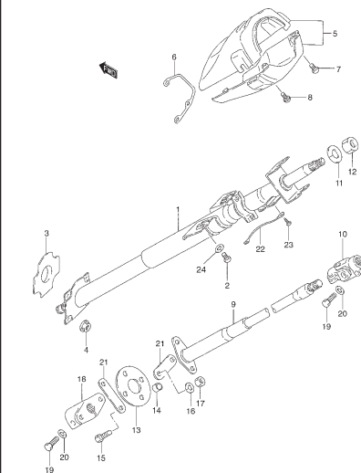
FIG. 54 COLUMNA DIRECCION
