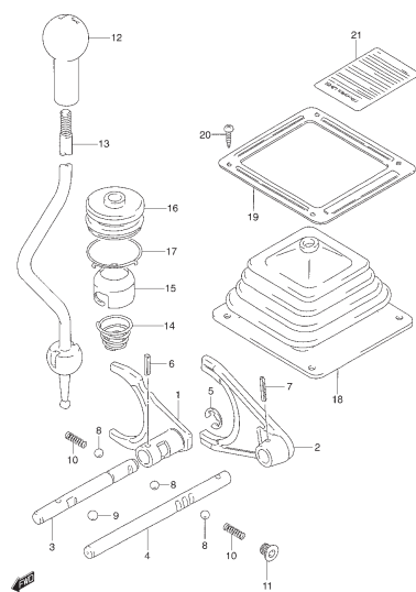
FIG. 32 PALANCA TRANSFERENCIA
