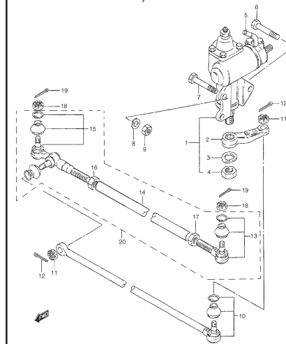
FIG. 56 CAJA DIRECCION (W/DIRECCION ASISTIDA)
