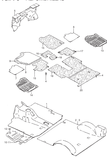
FIG. 79 ALFOMBRILLAS
