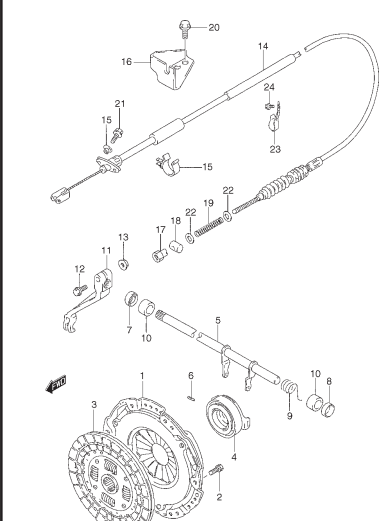
FIG. 23 EMBRAGUE
