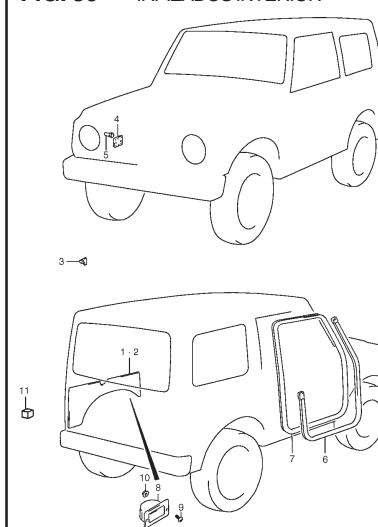
FIG. 80 TAPIZADOS INTERIOR
