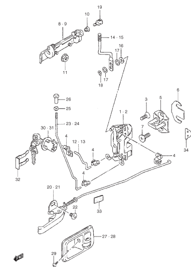
FIG. 88 CERRADURA PUERTA DELANTERA
