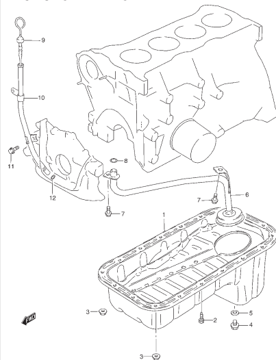
FIG. 5 CARTER ACEITE
