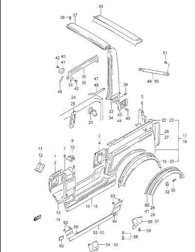
FIG. 70 PANELES LATERALES (J)
