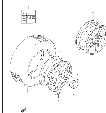
FIG. 52 NEUMATICO/LLANTA
