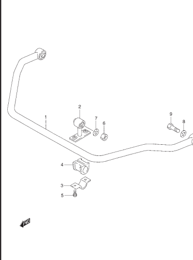
FIG. 47 BARRA ESTABILIZADORA
