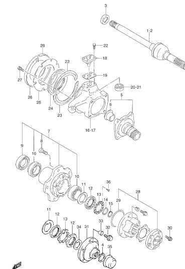
FIG. 48 EJE DELANTERO
