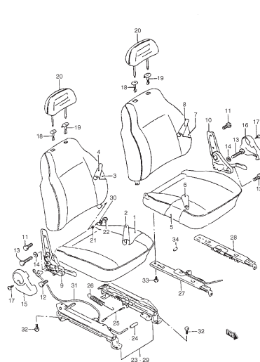
FIG. 94 ASIENTO DELANTERO
