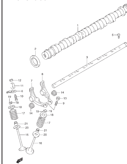
FIG. 8 CIGÜENAL
