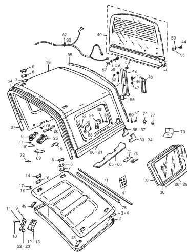
FIG. 85 TECHO DE FIBRA
