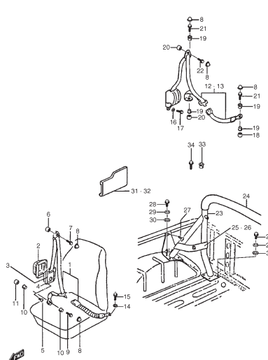
FIG. 96 CINTURONES DE SEGURIDAD
