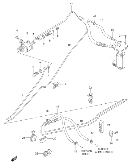
FIG. 17 CIRCUITO DE ALIMENTACION
