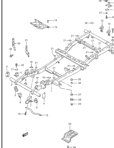
FIG. 64 CHASIS
