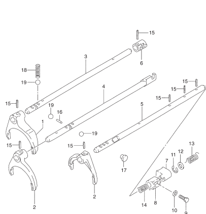
FIG. 26 HORQUILLAS SELECTORAS
