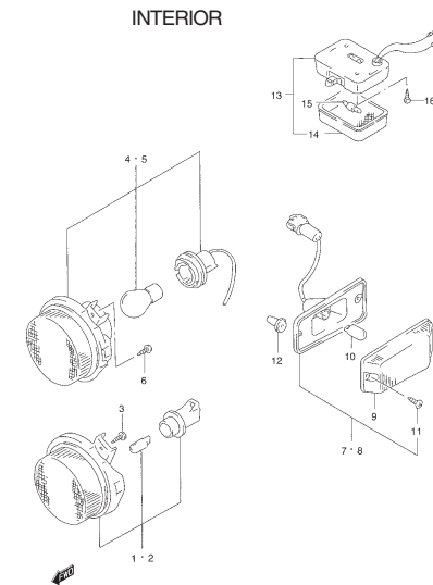
FIG. 40 PILOTO DELANTERO Y LUZ INTERIOR
