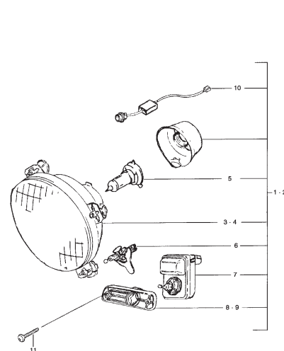
FIG. 39 FARO
