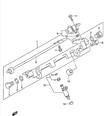
FIG. 13 TUBERIA DE ALIMENTACION
