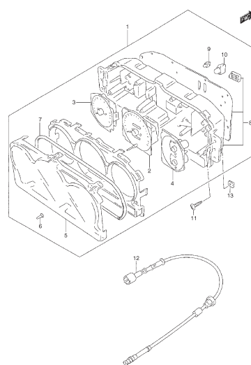
FIG. 38 PANEL COMBINADO
