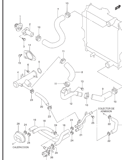
FIG. 20 MANGUITOS DE AGUA
