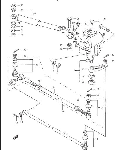
FIG. 55 CAJA DIRECCION (N/DIRECCION ASISTIDA)
