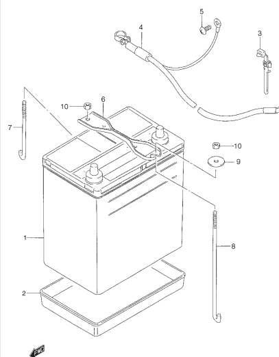
FIG. 37 BATERIA
