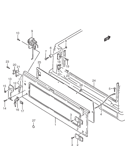
FIG. 89 PUERTA TRASERA (J)
