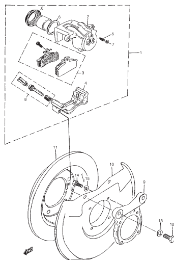
FIG. 61 FRENO DELANTERO
