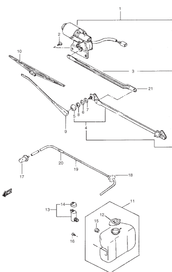
FIG. 45 LIMPIAPARABRISAS DELANTERO
