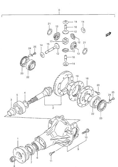
FIG. 29 DIFERENCIAL DELANTERO
