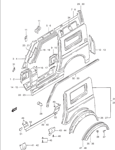
FIG. 71 PANELES LATERALES (V)
