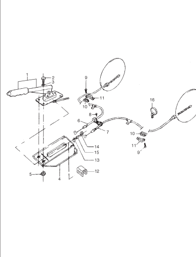
FIG. 63 FRENO DE MANO
