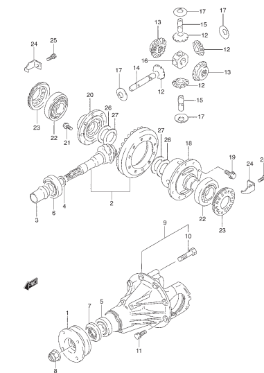
FIG. 30 DIFERENCIAL TRASERO
