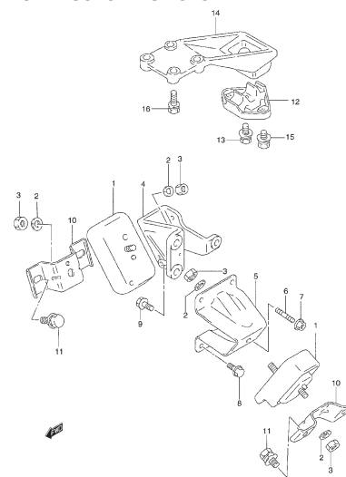
FIG. 7 SOPORTES MOTOR
