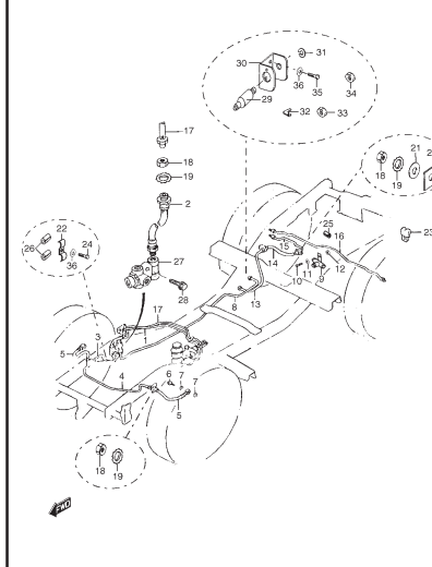
FIG. 64 CHASIS
