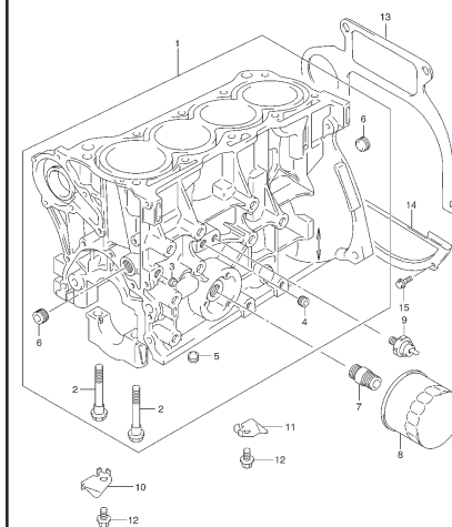
FIG. 4 BLOQUE CILINDROS
