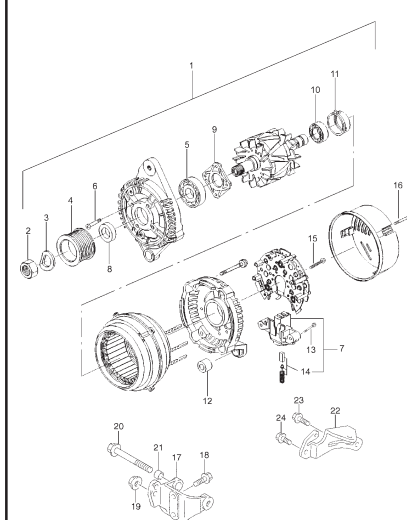
FIG. 36 ALTERNADOR
